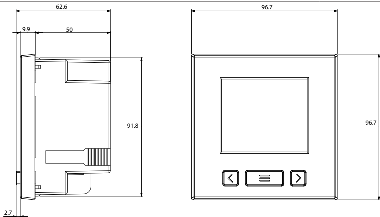
Dimensiones / Dimensions / Dimensiones / Dimensionen / Размеры / Dimensões
