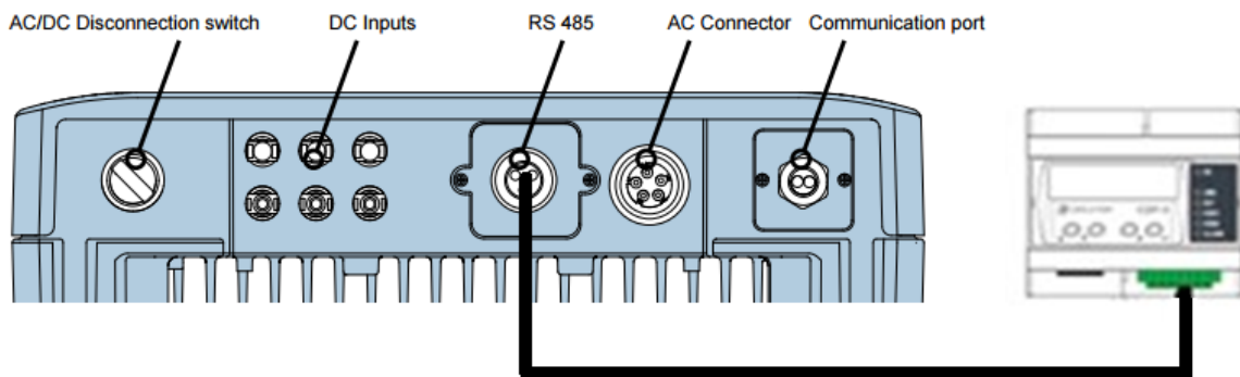
Figura 2: Conexión entre un CDP y un único inversor.
