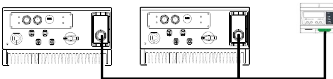
Figura 3: Conexión entre un CDP y varios inversor.
