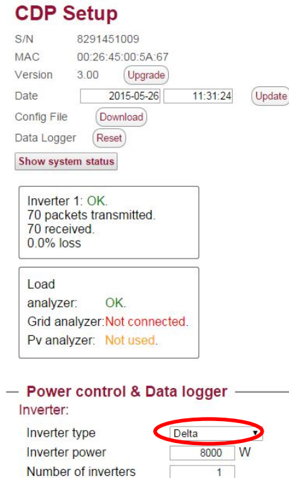
Figura 6: Página web de configuración del CDP.
