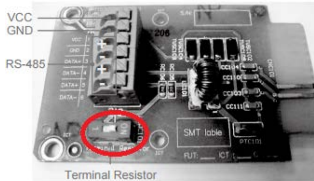
Figura 4: Terminal de final de bus.
