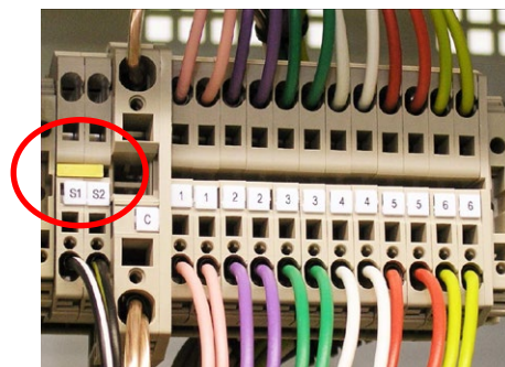
Fig. 5-3.- Terminales de conexión del TC
