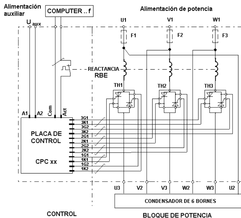
Fig. 4-4 .- Esquema básico de conexión de la CPCxx al bloque de potencia
