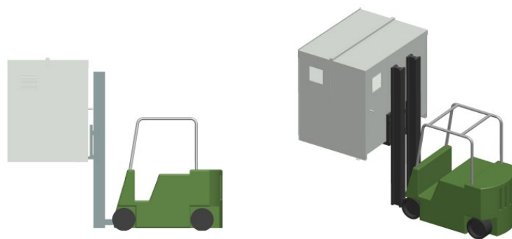
Fig. 3-2 .-Descarga con carretilla elevadora
