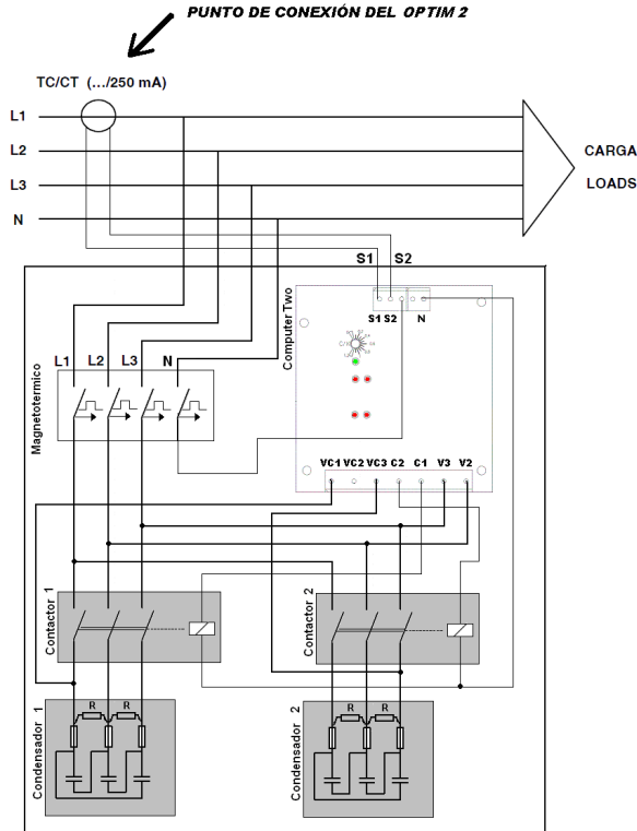
Fig. 3 Esquema conexión OPTIM 2
