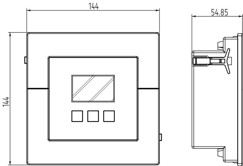
Figura 15: Dimensiones computer C Wi-Fi.
