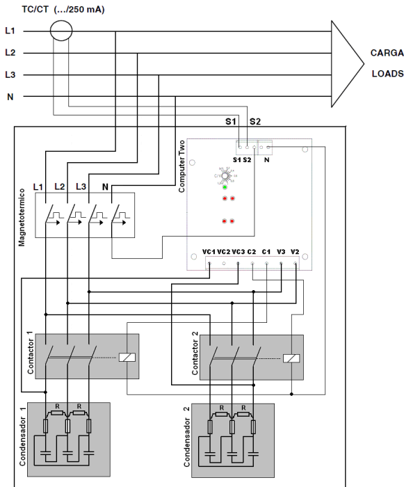
Fig. 3 Schéma connexion OPTIM 2
